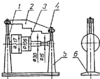
1 — опора; 2 — прижимная планка; 3 — цилиндр; 4 — гайка; 5 — опора; 6 — основание
