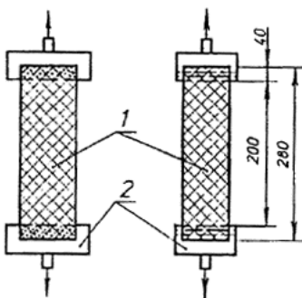
1 — образец; 2 — игольчатый зажим
