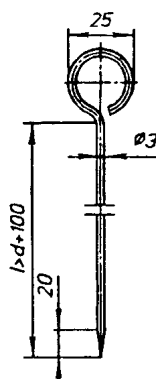
Рисунок А.2 — Игла
