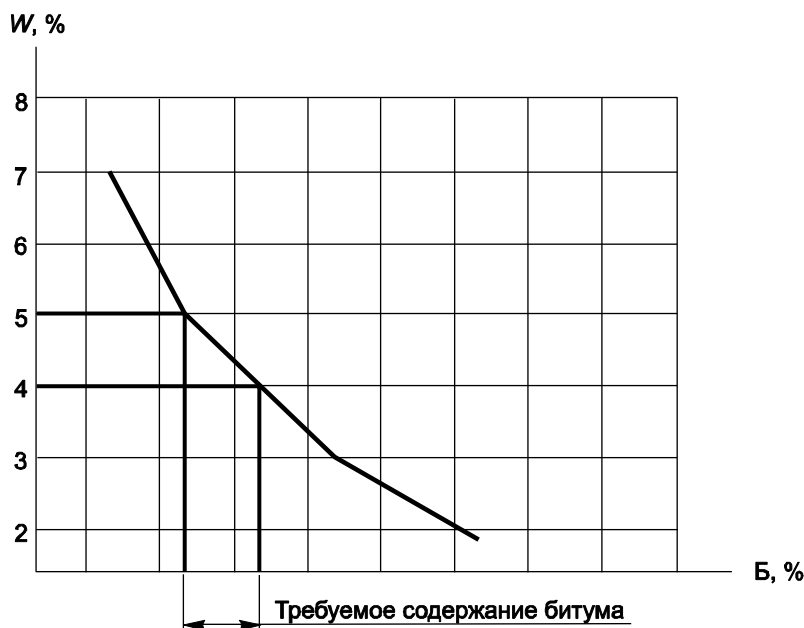
Рисунок 3 — Определение требуемого содержания битума
