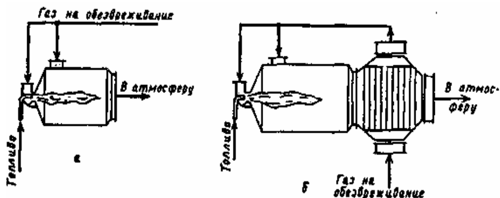
Рис. 7.4. Схемы термических нейтрализаторов промышленных отходящих газов: а - без теплообменника; б - с теплообменником
