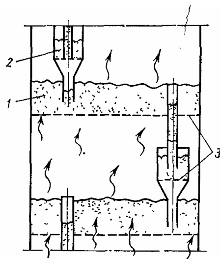
Рис. 4.10. Переточное устройство с дополнительным псевдоожиженным слоем адсорбента:
