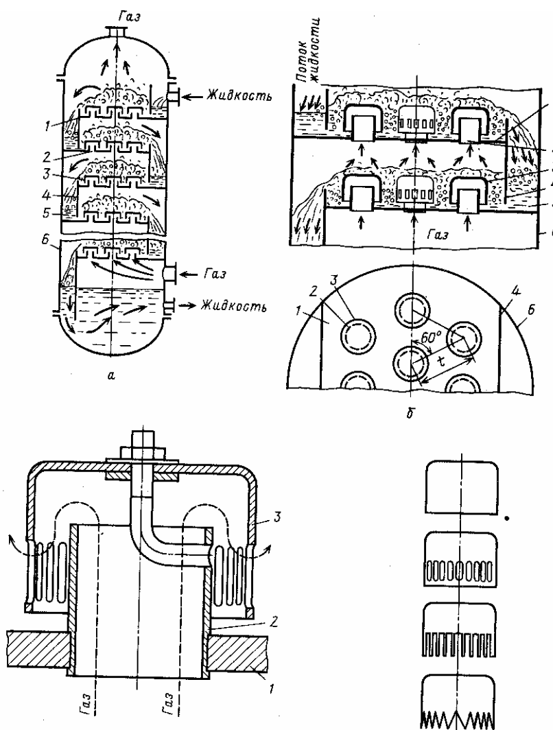
Рис. 3.7. Устройство колонны и колпачковых тарелок с капсульными колпачками:
