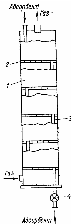
Рис. 4.8. Схема многоступенчатого адсорбера с псевдоожиженным слоем: 1 – псевдоожиженный слой; 2 – решетка; 3 – переток; 4 – затвор
