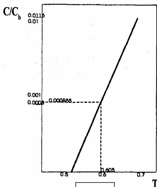
Рис. 4.18. Зависимость безразмерных концентраций C/C_n от безразмерного времени процесса T
