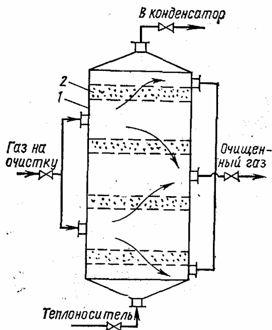
Рис. 4.1. Адсорбер полочного типа с неподвижными слоями адсорбента.
