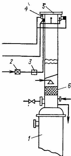
Рис. 7.2. Установка для факельного сжигания газообразных отходов, смонтированная на реакторе:
