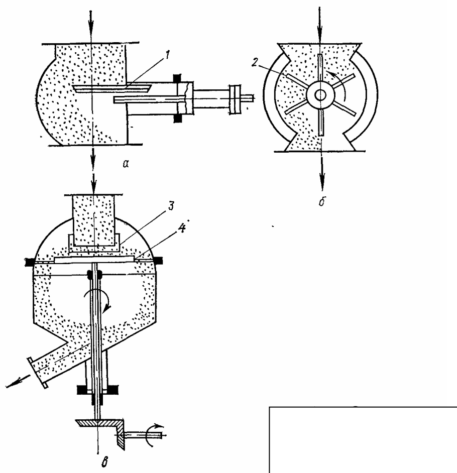
Рис. 4.14. Схемы типовых питателей: а – шиберный; б – секторный; в – тарельчатый; 1 – шибер; 2 – звездочка; 3 – регулирующий патрубкок; 4 – диск.
