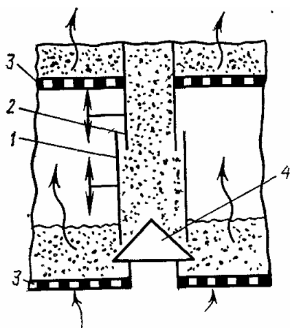
Рис. 4.11. Переточное устройство с коническим запорным устройством: 1, 2 – патрубки; 3 – решетки; 4 – конус
