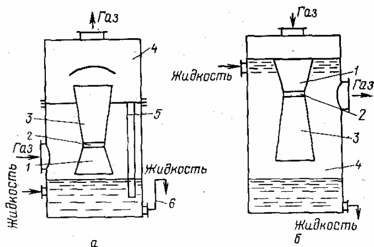
Рис. 3.16. Устройство бесфорсуночного абсорбера Вентури:
