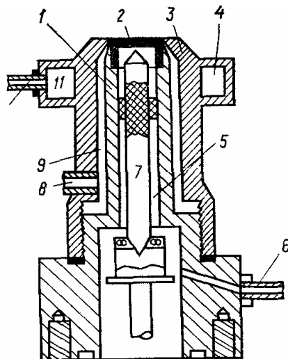
Рис. 7.7. Горелка для сжигания галогенсодержащих газов в атмосфере инертного газа:
