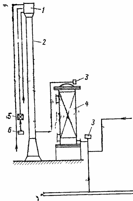
Рис. 7.3. Установка для факельного сжигания газов, содержащих ацетилен:
