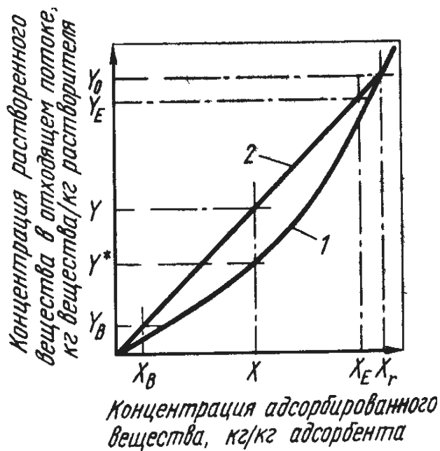
Рис. 4.17. Линия равновесия и рабочая линия в адсорбере с неподвижным слоем
