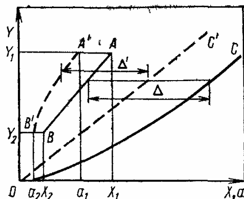
Рис. 3.26. Построение псевдорабочей и псевдоравновесной линии на диаграмме Y - X ( AB – рабочая линия; A'B' – псевдорабочая линия; OC – линия равновесия; OC' – псевдоравновесная линия)
