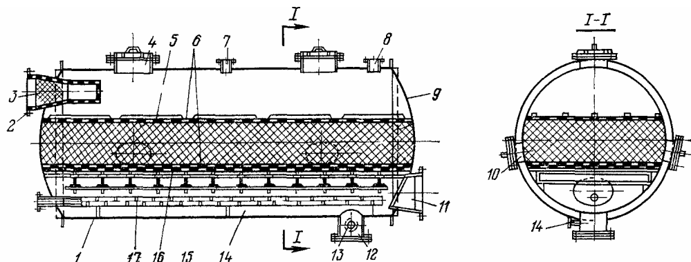
Рис. 4.5. Горизонтальный адсорбер:
