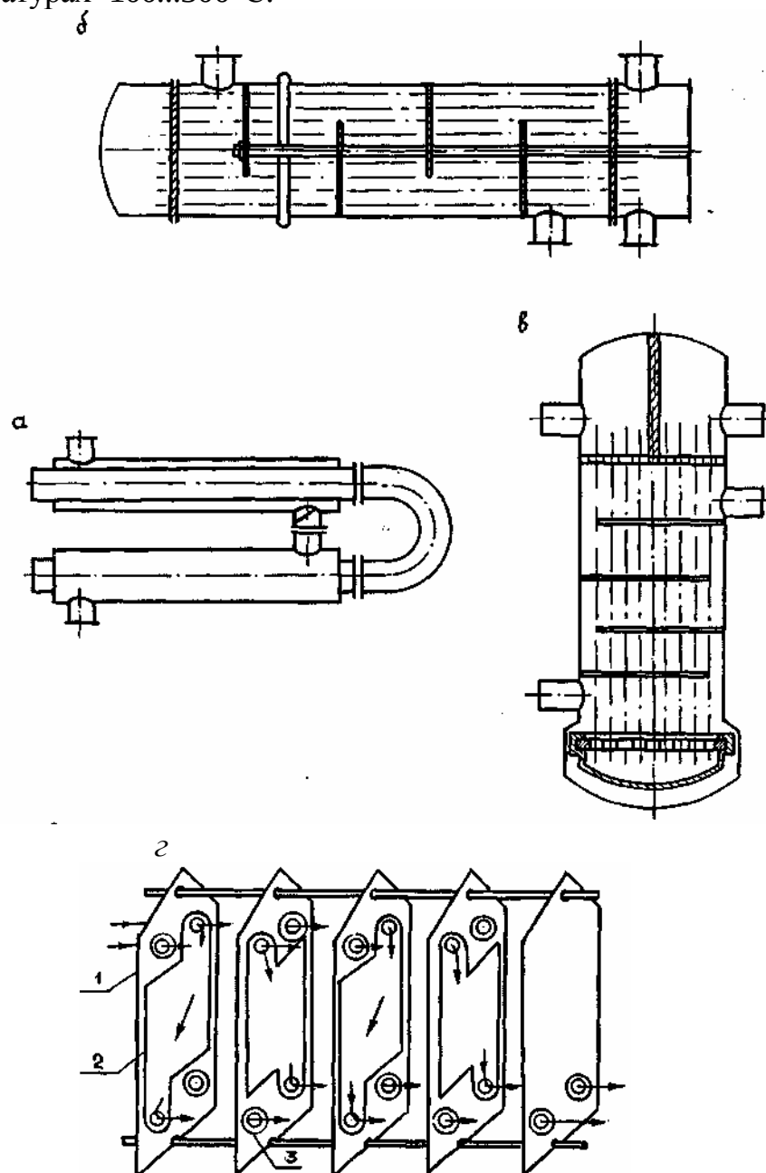
Рис. 5.1. Конструкции теплообменников-конденсаторов.
