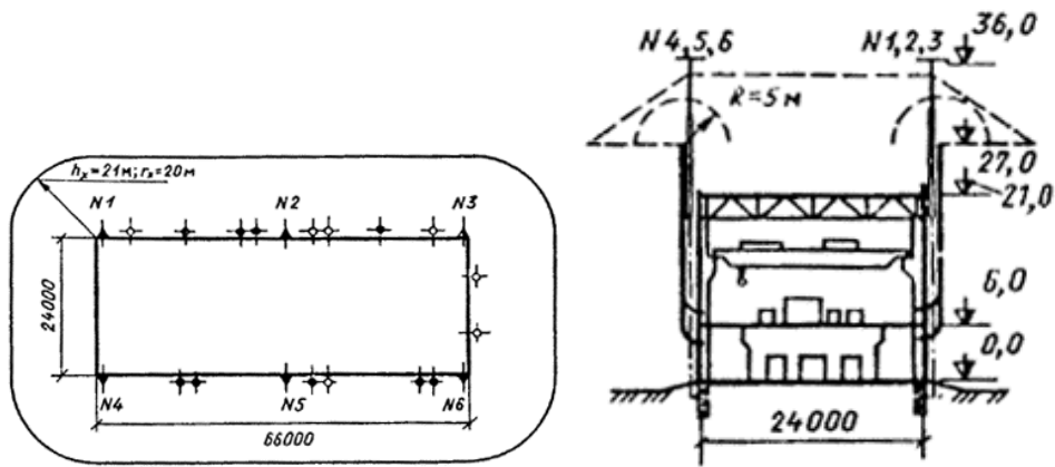
Рис. П4.6. План цеха компрессии азотоводородной смеси (относится к взрывоопасным с зоной класса В-1а) : Условные обозначения: \Delta \blacktriangle — стержневой молниеотвод (№ 1-6); —.—.—- токоотводящая металлическая полоса; O — газоотводные трубы для отвода в атмосферу газов невзрывоопасной концентрации; • — то же взрывоопасной концентрации
